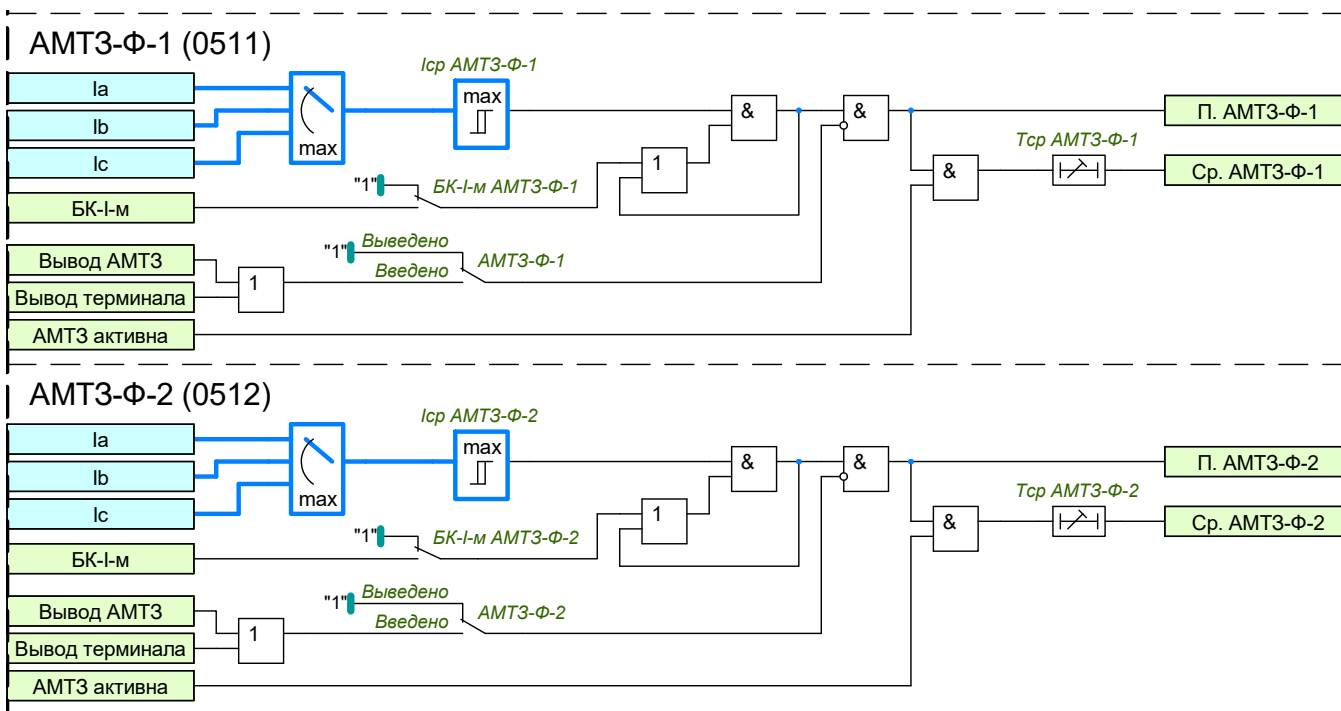
Рисунок 1.26 – Функциональная схема ступеней АМТЗ-Ф-1(2)
