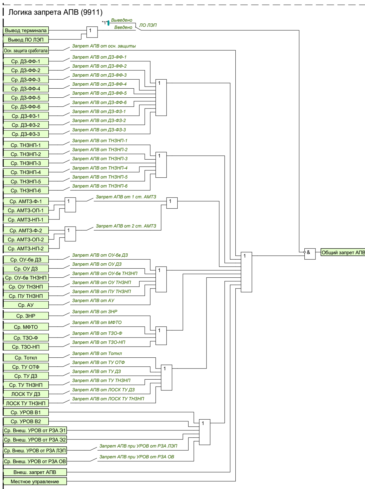
Рисунок 1.44 – Функциональная схема общего запрета АПВ
