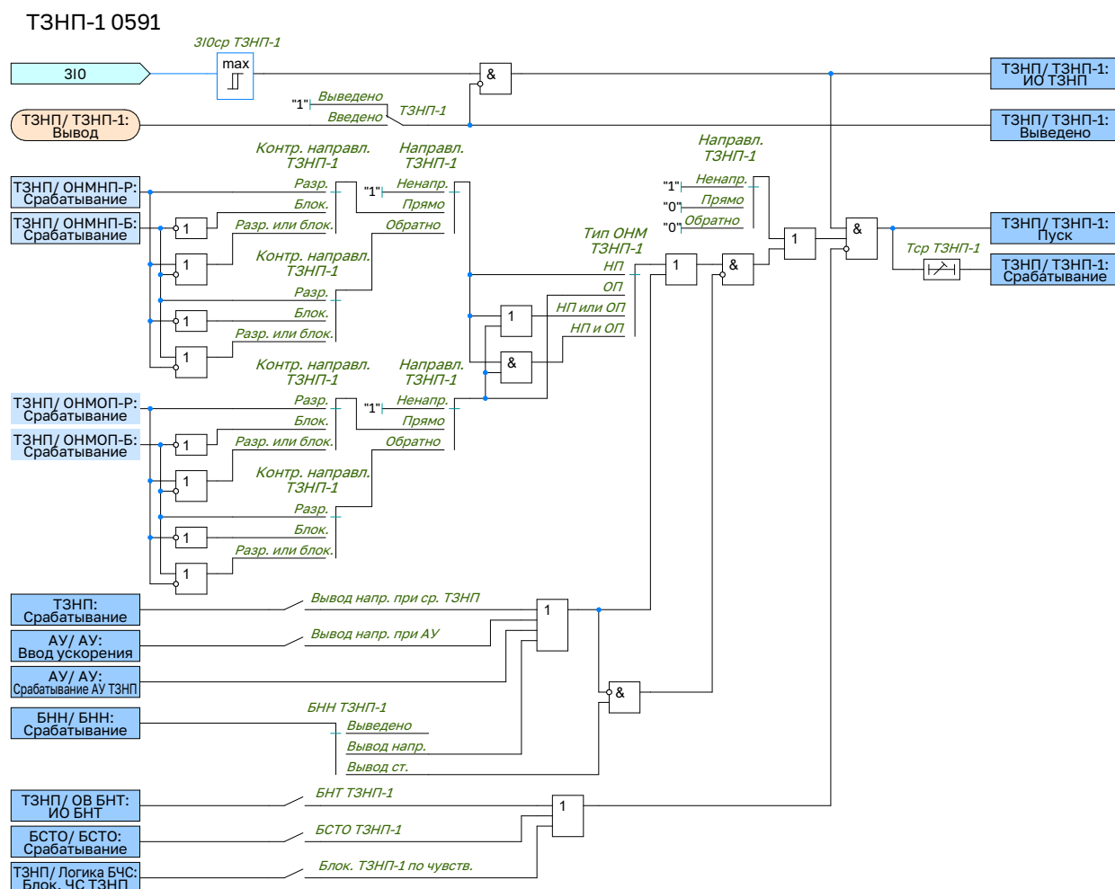
Рисунок 1.19 – Функциональная схема ступени ТНЗНП-1
