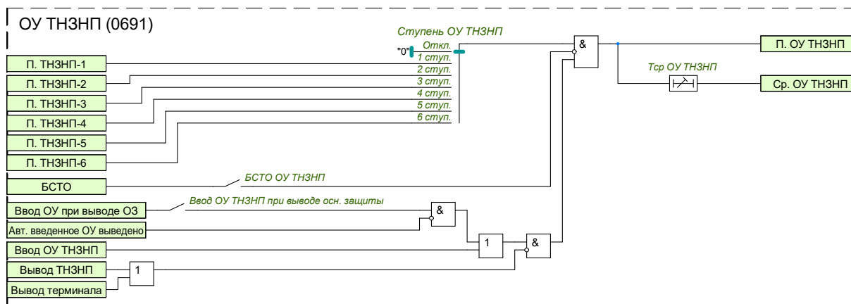
Рисунок 1.22 – Функциональная схема ОУ ТНЗНП
